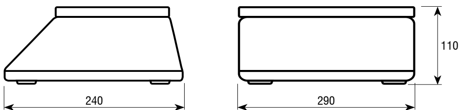
Dimensiones (mm)
